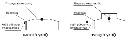
Σχ. 5. Παραδειγματική ρύθμιση του καπνοσύρτη
