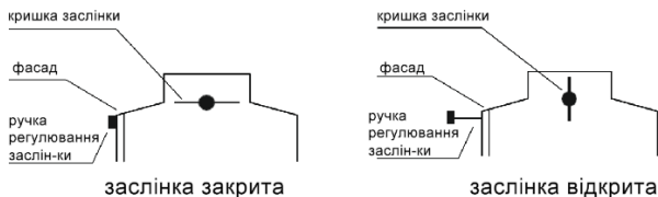
Рис. 5. Приклад регулювання заслінки
