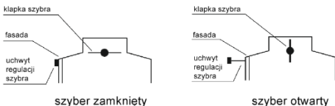
Rys. 5. Przykładowa regulacja szyby.
