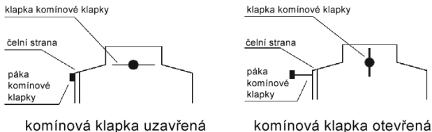
Obr. 5. Příklad regulace komínové klapky
