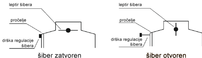
Crtež 5. Primjer regulacije šibera
