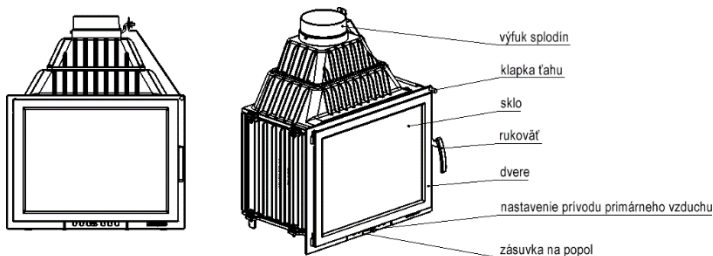
Obr. 1. Schéma krbovej vložky.
