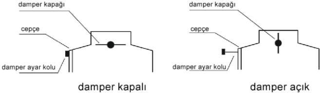
Şek. 5. Bir damper ayarı örneği
