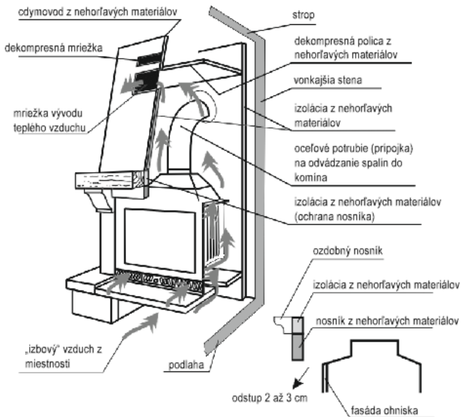
Obr. 2. Názorný spôsob inštalovania krbových vložiek.
