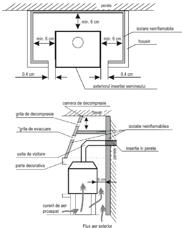
Fig. 3. Exemflu de instalare a unei insertii de semineu-vedere laterala
