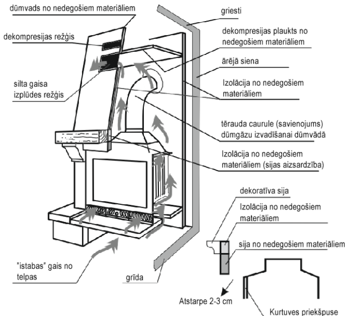
Att. 2 Piemērs, kā uzstādīt kamīna ieliktnus.
