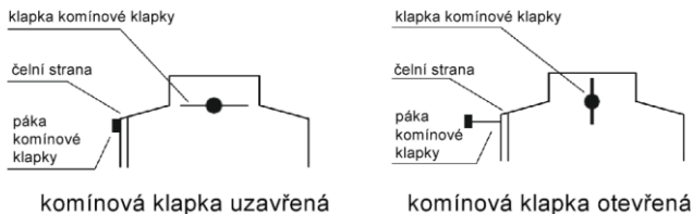
Obr. 5. Příklad regulace komínové klapky
