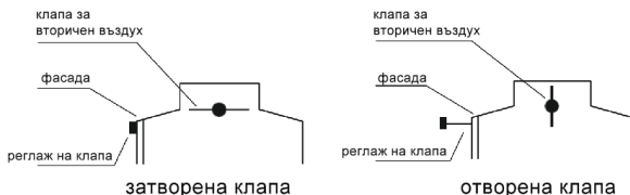
Фиг. 5. Пример за релгаж на клапа
